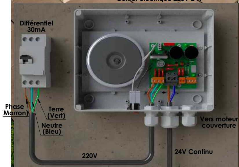
Coffret électrique 220V 24V
